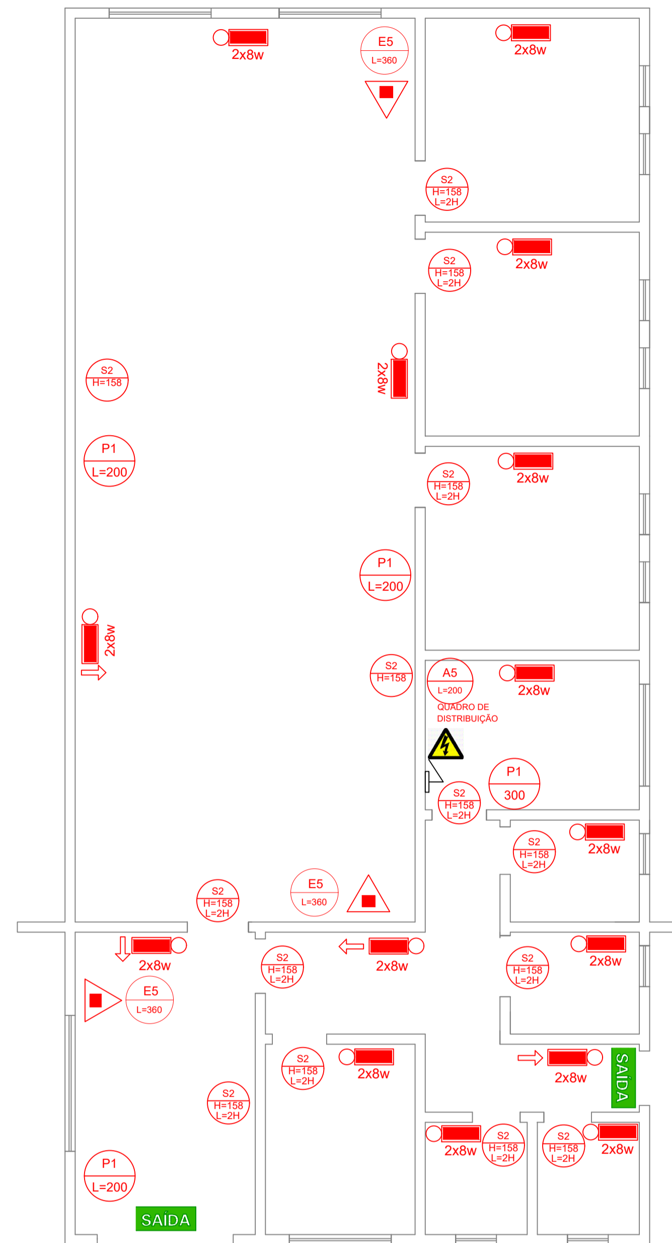
PLANTA BAIXA - PROJETO DE PROTEÇÃO CONTRA INCÊNDIO E PÂNICO ESCALA 1:50
