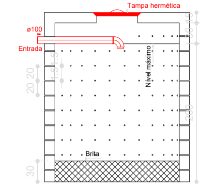
SUMIDOURO CORTE - ESC. 1:50
