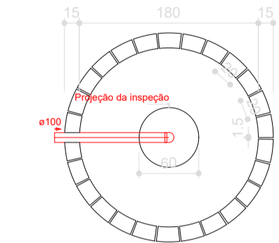
SUMIDOURO PLANTA BAIXA - ESC. 1:50
